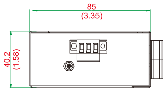
顶视图
