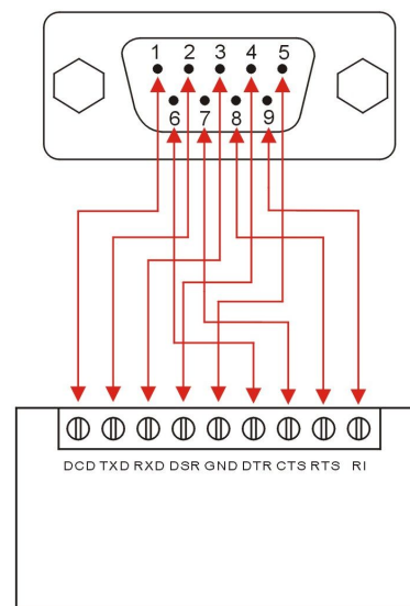
RS-232设备
