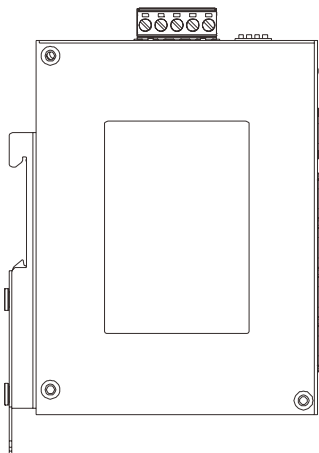
右侧视图
