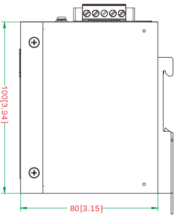
左侧视图
