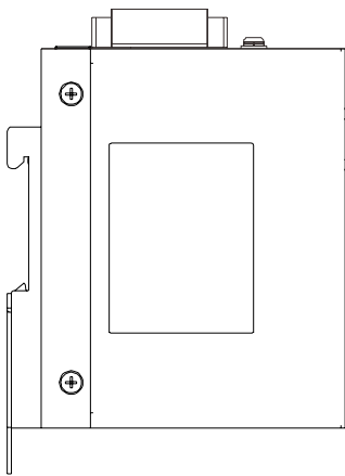
右侧视图
