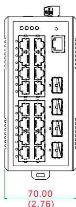
前视图
