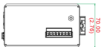
顶视图
