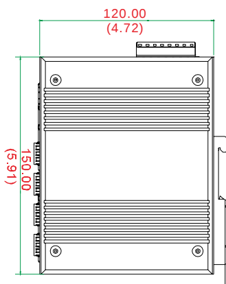
顶视图
