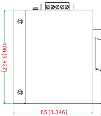
左侧视图
