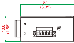
顶视图
