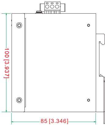
左侧视图
