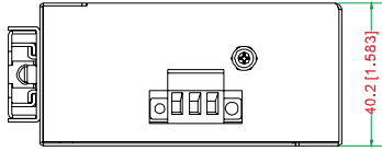
顶视图
