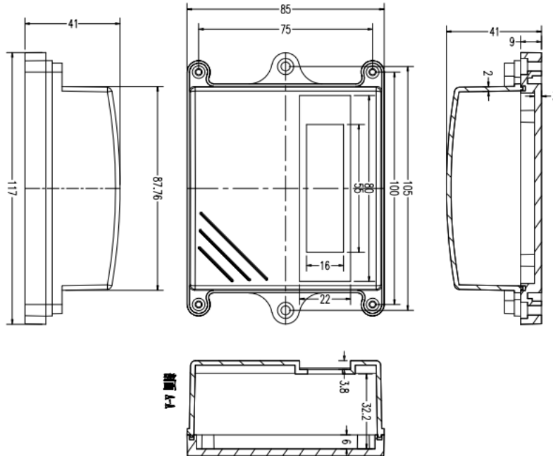
结构尺寸图
