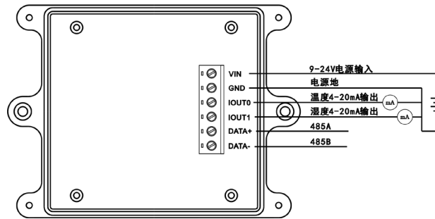
接线示意图
