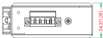
顶视图
