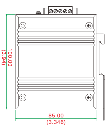
左侧视图
