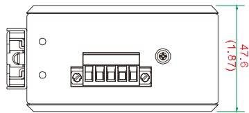
顶视图
