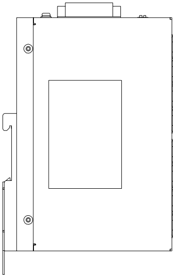
右侧视图
