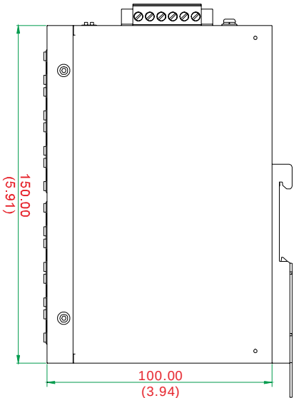
左侧视图
